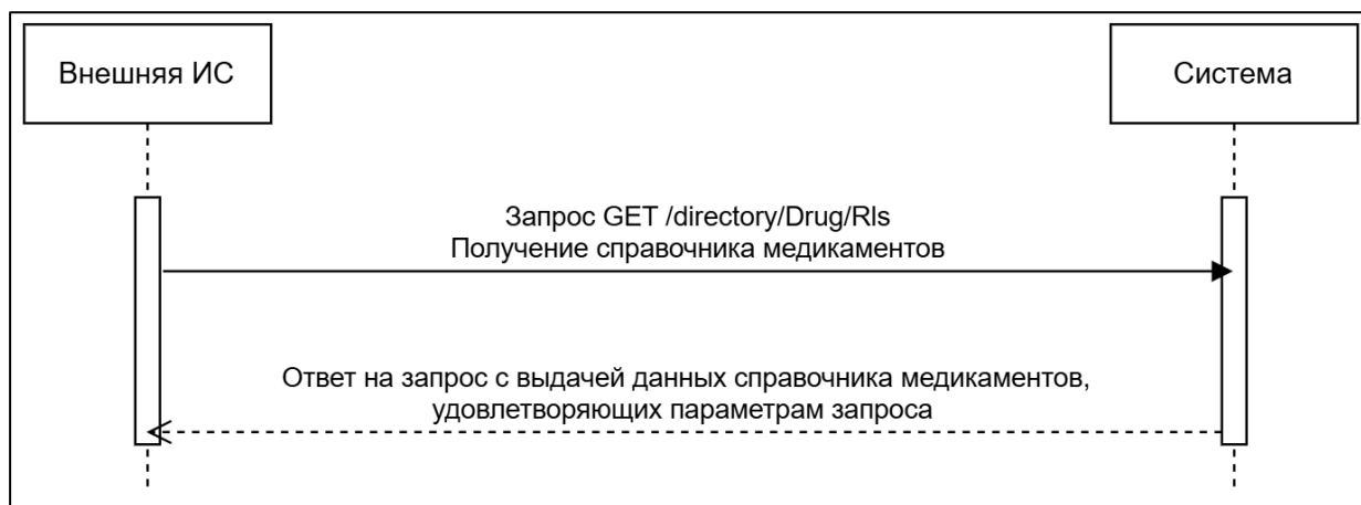
Рисунок 10 – Схема взаимодействия в части передачи справочника медикаментов
