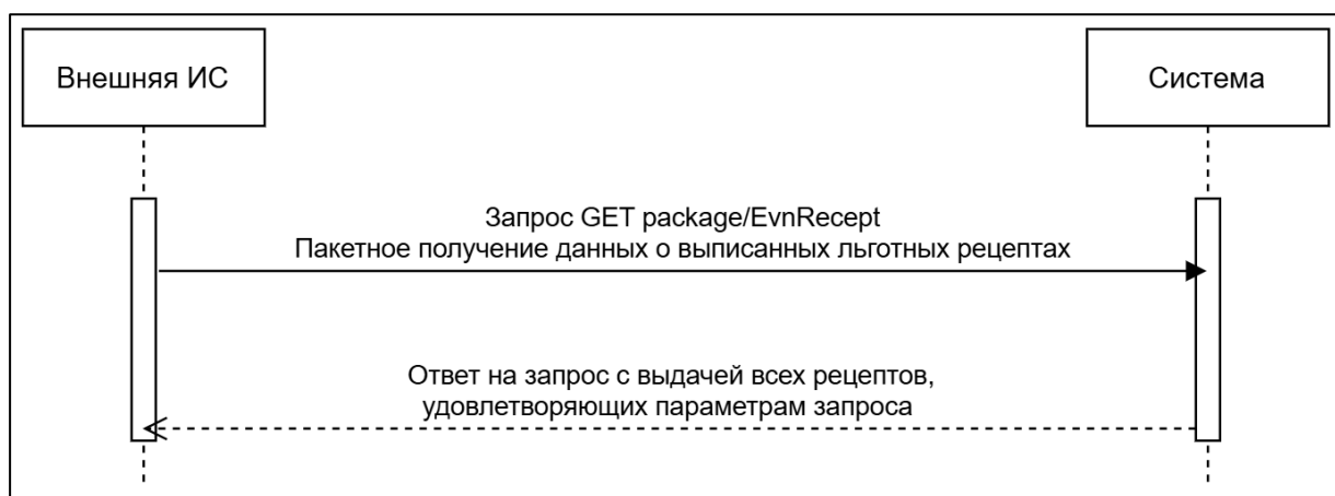
Рисунок 6 – Схема взаимодействия в части пакетной передачи данных о выписанных льготных рецептах
