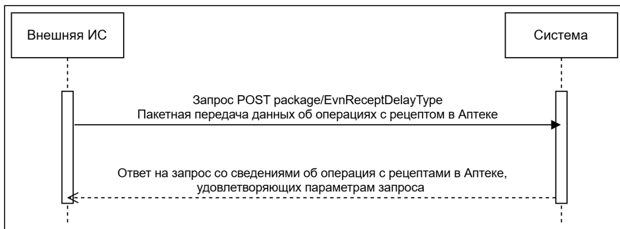
Рисунок 8 – Схема взаимодействия в части пакетного получения данных об операциях с рецептом в аптеке
